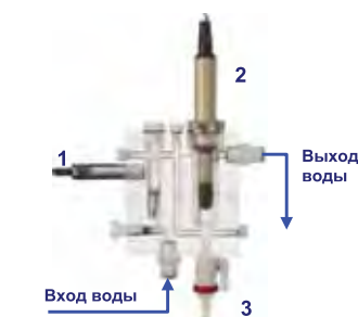
Рис. 131. Измерительная ячейка AQC-D6.
