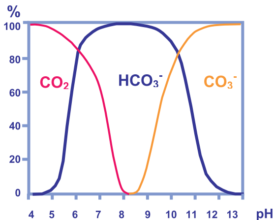
Рис. 5. Зависимость форм угольной кислоты от pH
