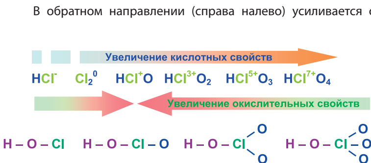
Рис. 72. Изменение кислотных и окислительных свойств кислородсодержащих соединений хлора.
