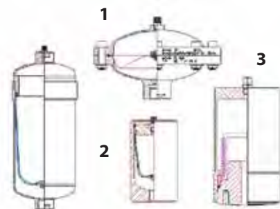
Рис. 107. Демпфер пульсаций.
