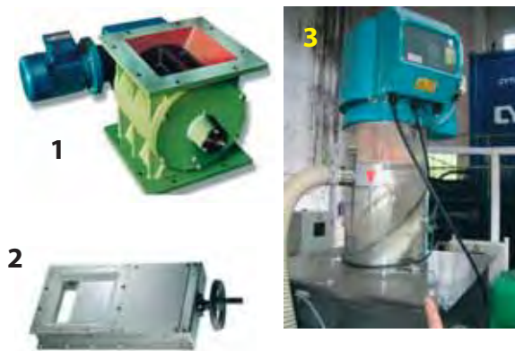
Рис. 46. Устройства для загрузки сухого полиэлектролита в шнековый дозатор установки Polydos - 412.
