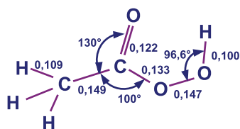
Рис. 69. Структурная формула надуксусной кислоты
