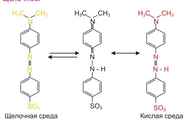
Рис.26. Метиловый оранжевый
