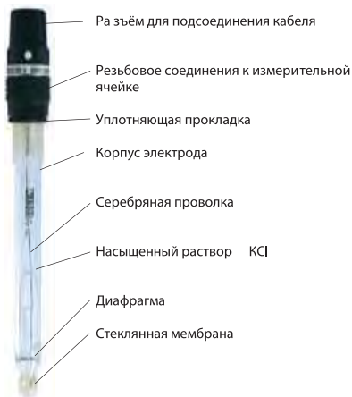
Рис. 14. Grundfos Alldos pH электрод 312-100
