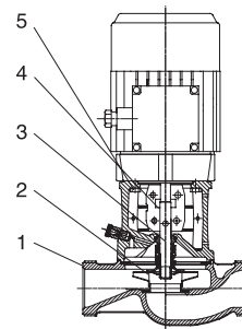
Разрез насоса TP серии 100 (с резьбовым присоединением)
