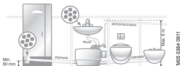
Рис. 23 Пример монтажа
