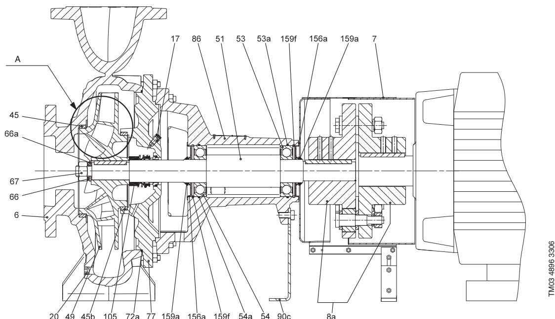
Рис. 4 Насос NK в разрезе
