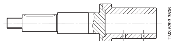
Рис. 14 Удлинитель вала типа 2
