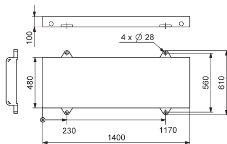
Рама-основание
