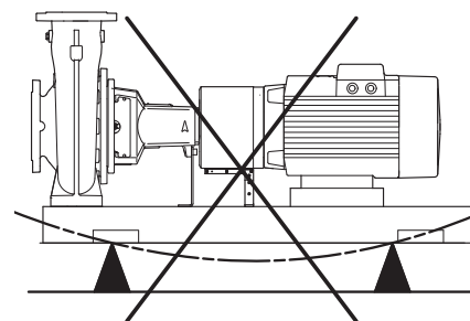
Рис. 25 Неправильный фундамент
