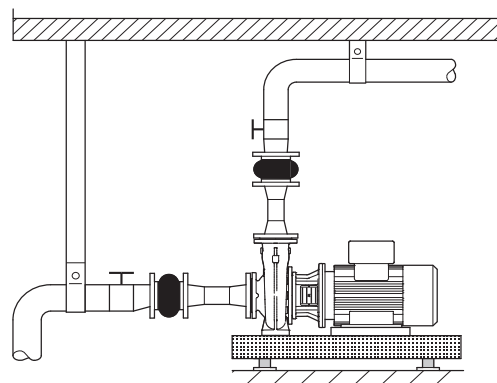
Рис. 29 Монтаж трубопровода
