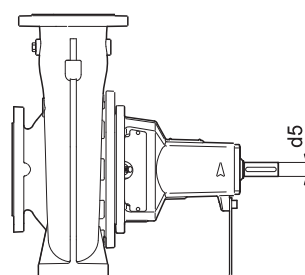
Рис. 20 Диаметр конца вала d5
