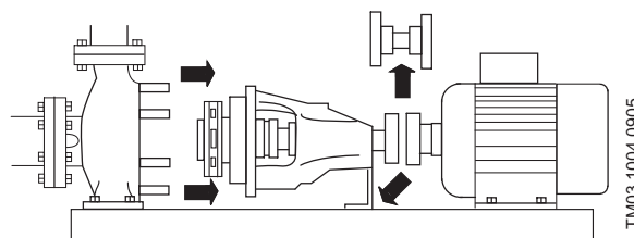
Рис. 2 Демонтаж электродвигателя насоса NK
