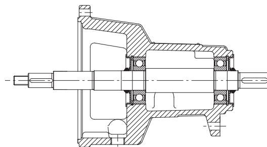
Рис. 9 Фонарь насоса и вал
