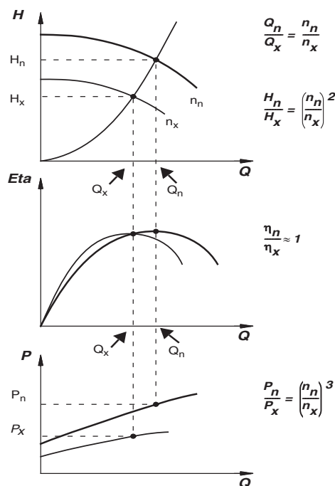
Рис. 32 Уравнения подобия
