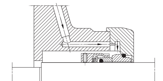
Рис. 11 Неразгруженное уплотнение AQAE для высоких давлений
