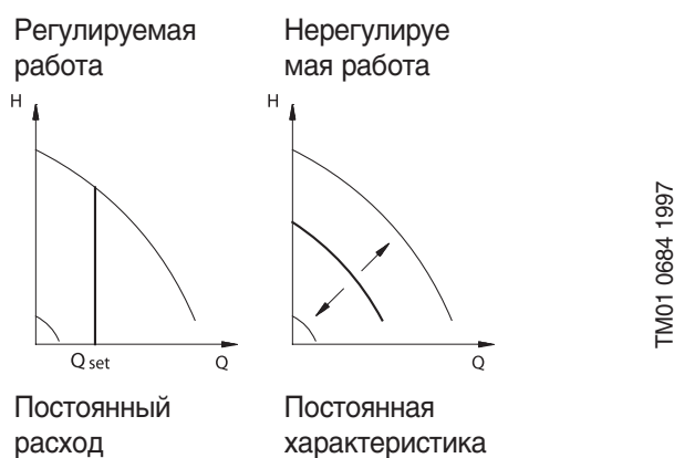
Рис. 14 Регулируемый и нерегулируемый режимы эксплуатации
