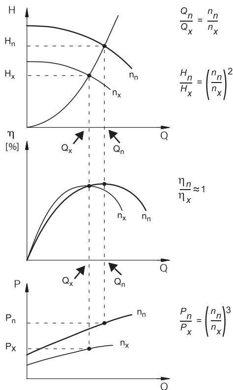
Рис. 34 Уравнения подобия
