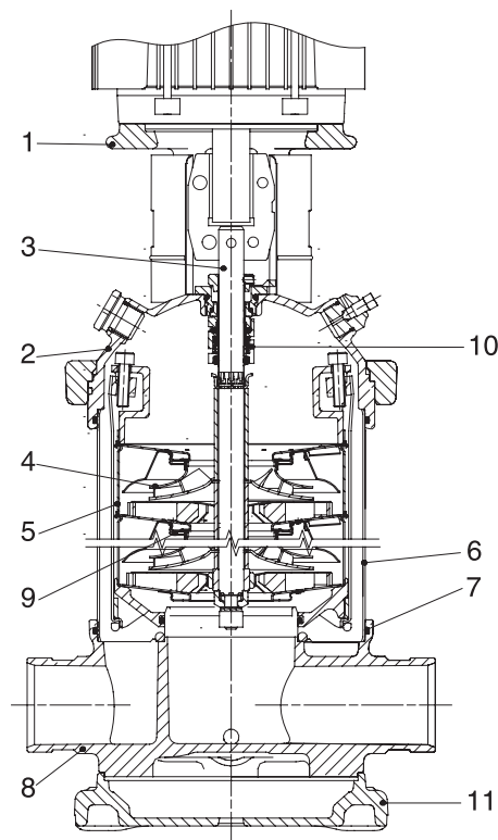
Чертеж насосов CRN 3, 5, 10, 15, 20 SF в разрезе
