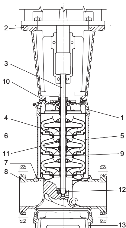
Чертеж насоса CR(N) в разрезе
