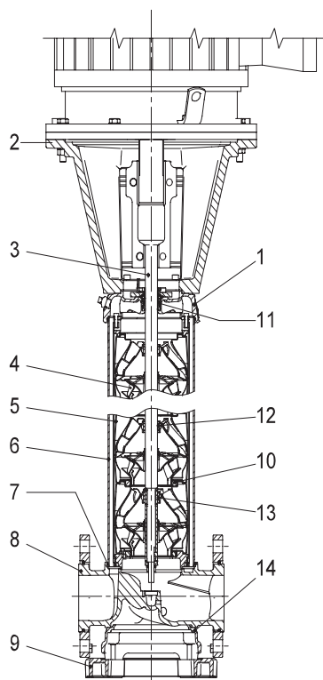
Чертеж насоса CR(N) в разрезе
