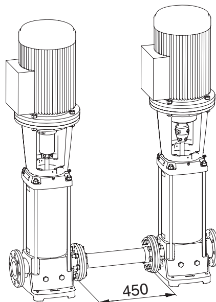
Питательный насос CRN, соединительная труба и насос высокого давления CRN SF
