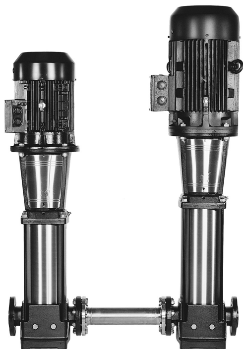
2-х CR, CRN-система сдвоенных насосов
