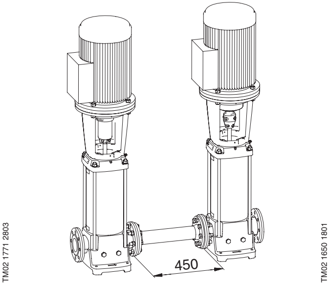
Питательный насос CRN, соединительная труба и насос высокого давления CRN SF
