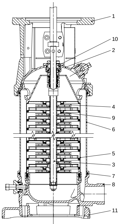
Чертеж насосов CRNE 1 и 3 HS в разрезе
