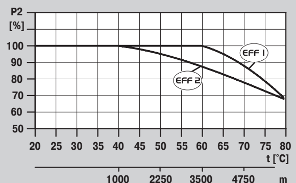
Падение мощности электродвигателя в зависимости от температуры и высоты над уровнем моря
