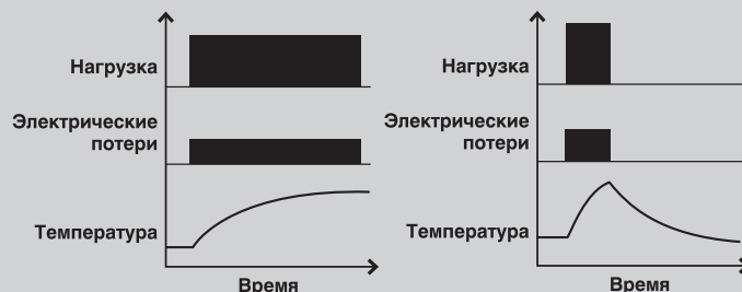
Тип рабочего цикла (нагрузки) S1 – непрерывный режим
