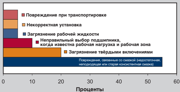
Причины повреждений в роликовых подшипниках
