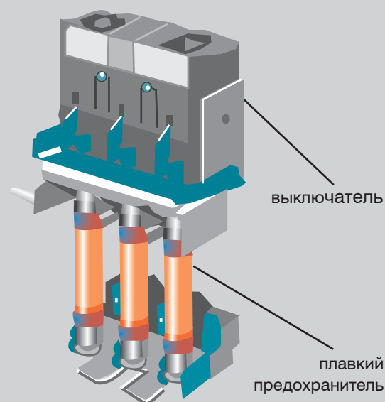
Плавкий предохранительный выключатель
