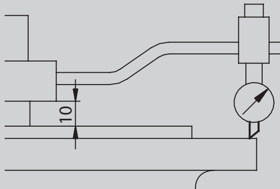
Перпендикулярность установочной поверхности фланца к валу
