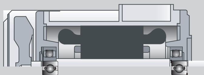
Блок подшипников с плавающим подшипником и пружинной шайбой на стороне без привода и зафиксированным шарикоподшипником с глубокими дорожками качения на стороне с приводом
