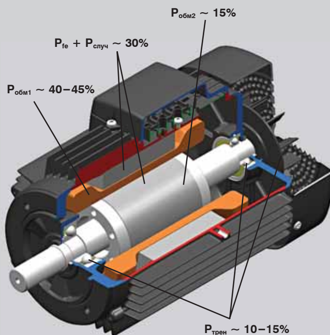
Распределение потерь в индукционном электродвигателе
