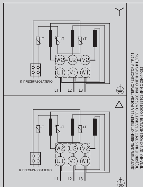
Типичная схема электрических соединений
