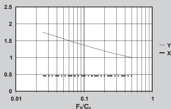
X и Y в зависимости от F_a/C_0 допустимый зазор при эксплуатации
