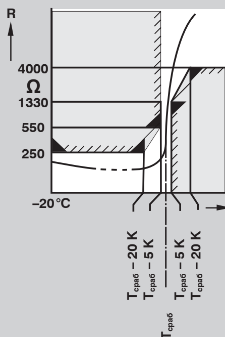
Критические значения характеристики сопротивление/температура для датчиков защиты электродвигателя.
