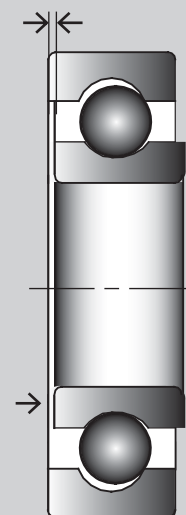
Осевой внутренний зазор
