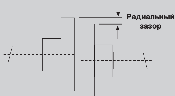
Радиальное согласование (концентричность) S_1
