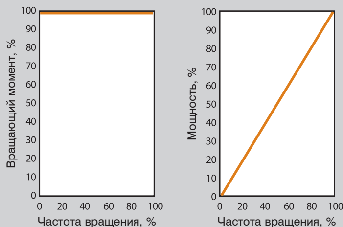
Постоянный вращающий момент независимо от скорости вращения
