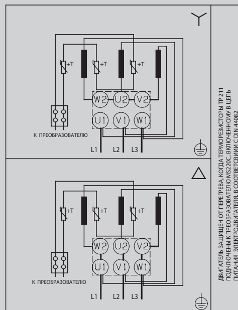
Схема подключения
