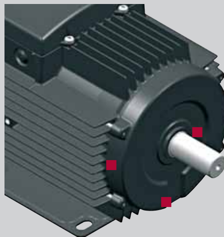
Дренажные отверстия на рисунке отмечены красными квадратами ■
