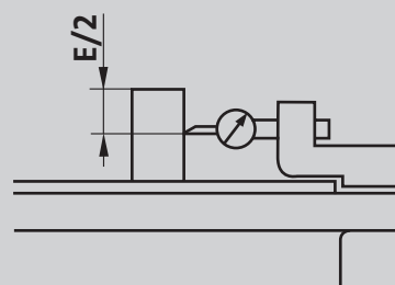
Эксцентricность вала электродвигателей B14/V18/B5/V1
