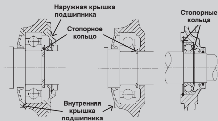
Схема установки зафиксированных DE-подшипников
