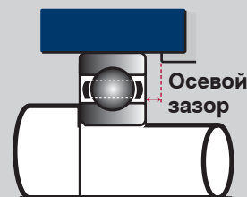
Плавающий подшипник
