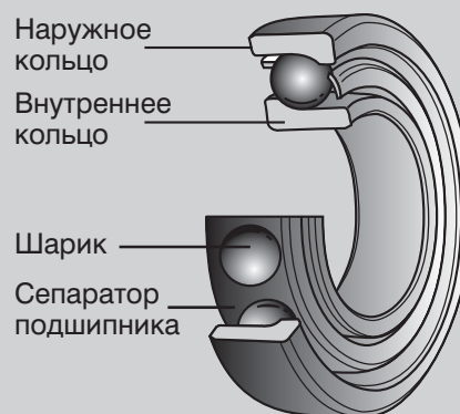
Радиально-упорный шарикоподшипник
