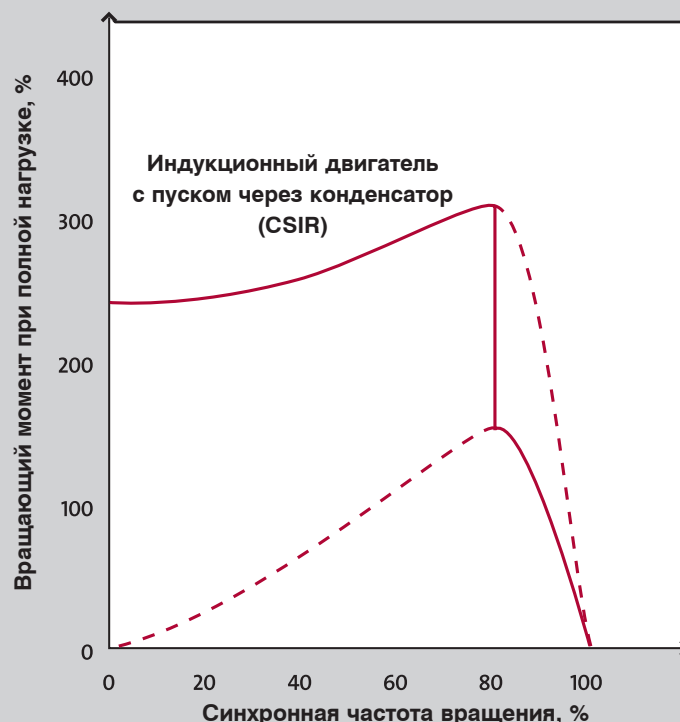
Электродвигатель CSIR. Схема электрических соединений и кривая соотношения момент/частота вращения
