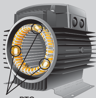
Три датчика РТС: по одному в каждой фазе
