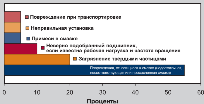
Причины разрушения подшипников качения
