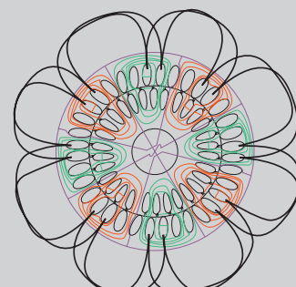
3-фазный, 8-полюсный электродвигатель
