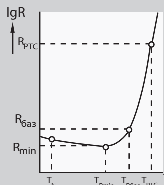
Сопротивление в зависимости от температурной характеристики терморезистора PTC (DIN 44081/44082)
