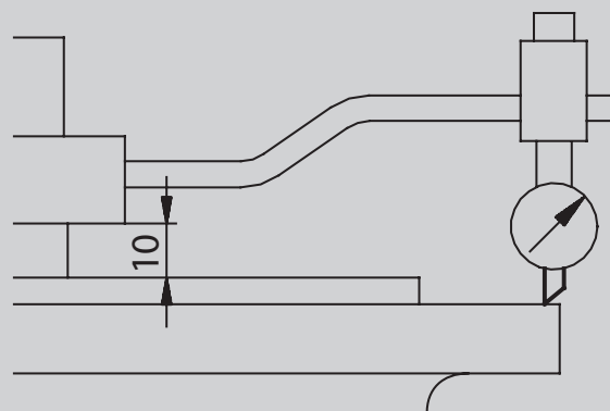
Взаимная перпендикулярность поверхностей вала и фланца
