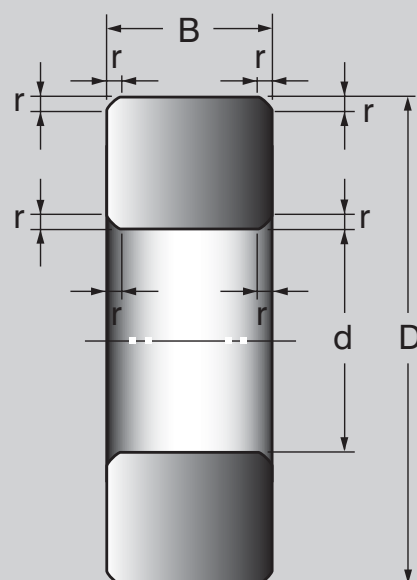
Габаритные размеры радиально-упорных подшипников
