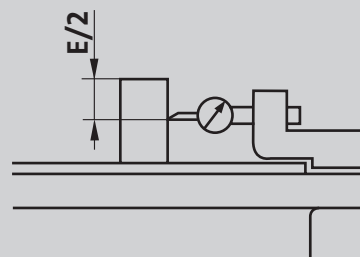
Эксцентриситет конца вала для электродвигателей B14/V18/B5/V1
