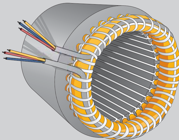
Статор
