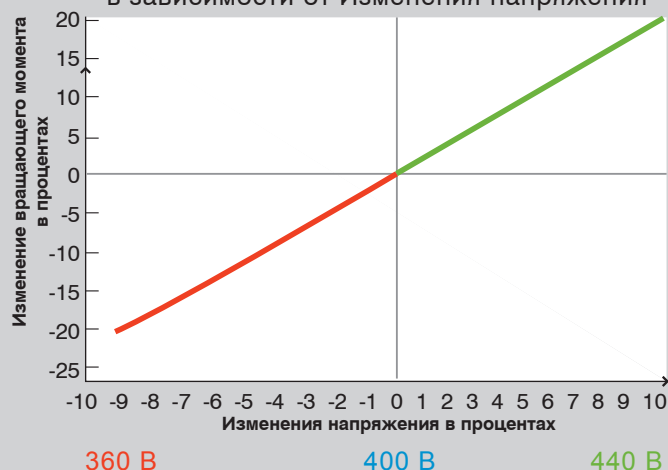
Изменение вращающего момента в зависимости от Изменения напряжения
