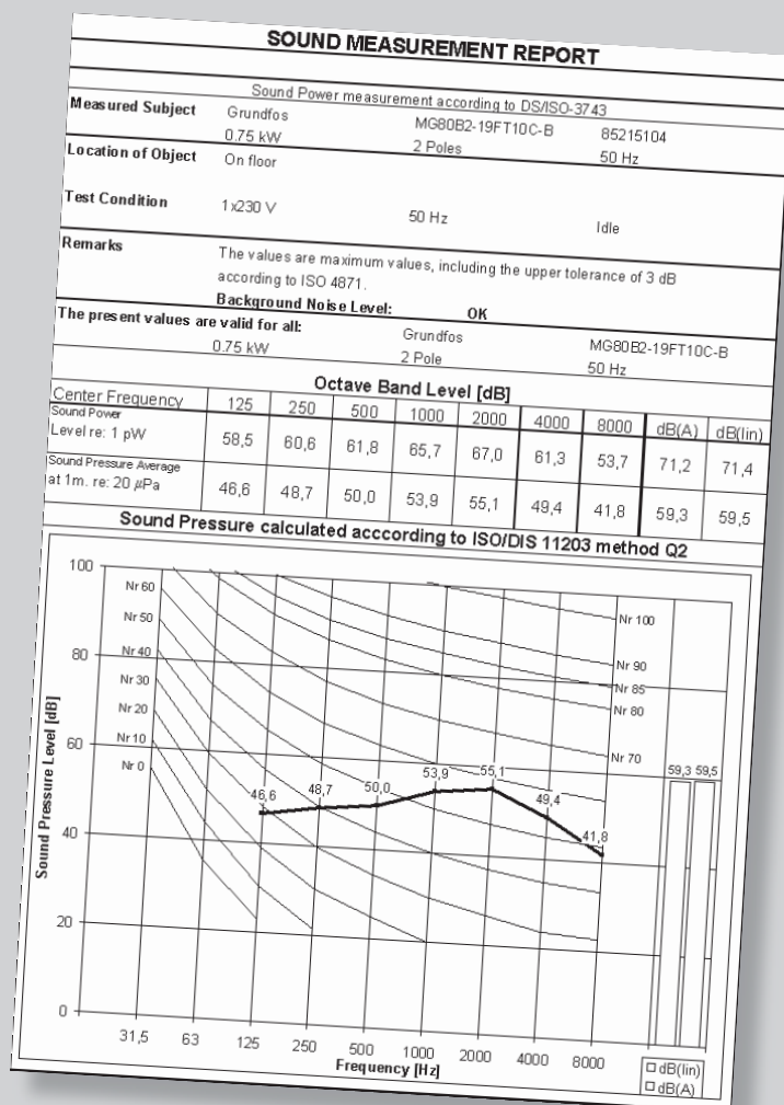
Отчёт Grundfos об измерении звука
