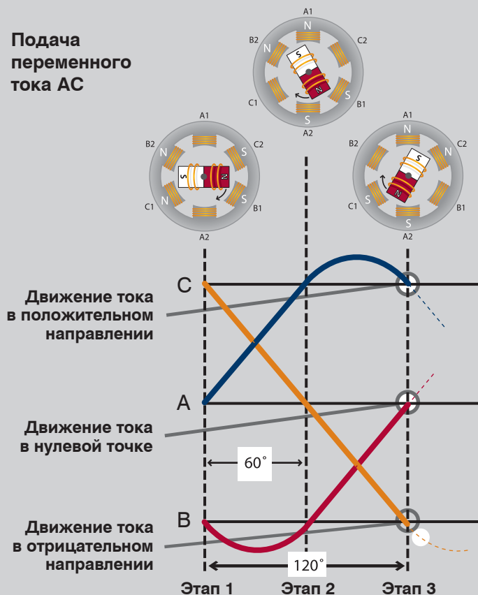
3-фазный, 2-полюсный электродвигатель
