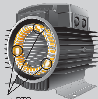
Три датчика РТС: по одному на каждой фазе
