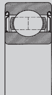
Шарикоподшипник с глубокими дорожками качения с металлическими стыковыми накладками. Известен как тип ZZ
