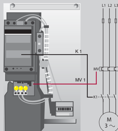
K 1 = Контактор MV 1 = Реле перегрузки
