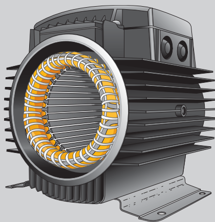
Статор в корпусе, подготовленный для сушки
