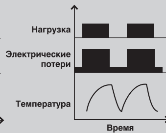
Тип рабочего цикла S6 – непрерывный режим с периодической нагрузкой
