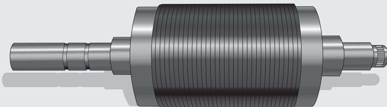
Обмотки проводников ротора изготовлены из алюминия
