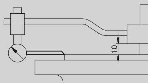
Концентricность центрирующего буртика вала
