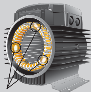
3 датчика ПТС; По одному на каждой фазе
