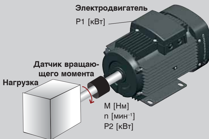
Измерения с использованием прямого метода
