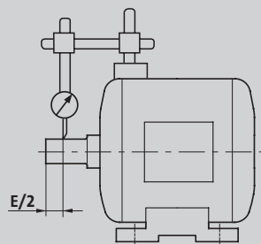
Эксцентricность вала электродвигателя B3
