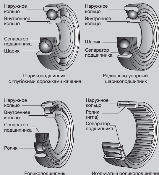
Различные типы шариковых и роликовых подшипников
