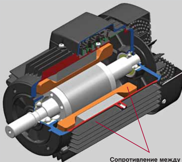
Измерение изоляции на «землю»
