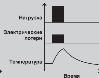
Тип рабочего цикла S2 – кратковременный режим работы
