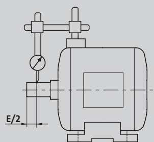
Электродвигатели с эксцентриситетом конца вала B3
