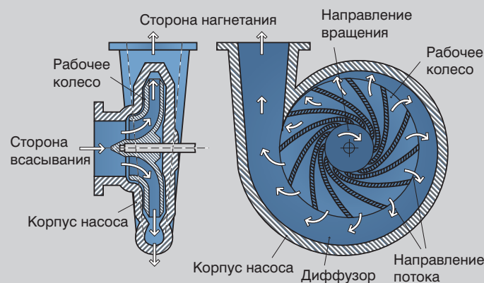
Центробежный насос, поперечный разрез
