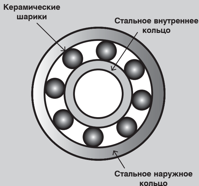
Гибридные подшипники
