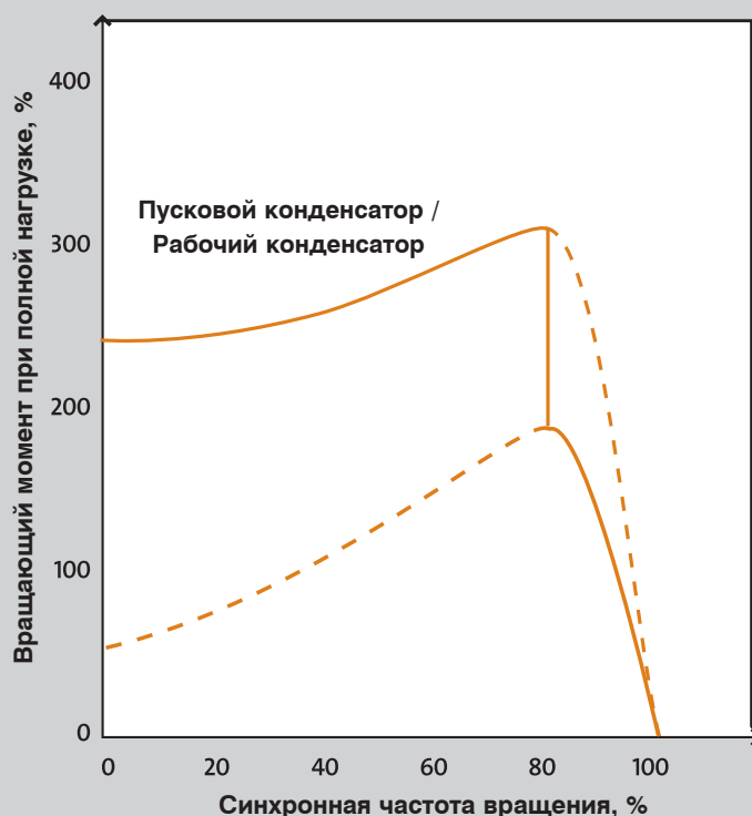
Электродвигатель CSCR. Схема электрических соединений и характеристика пускового момента/частота вращения
