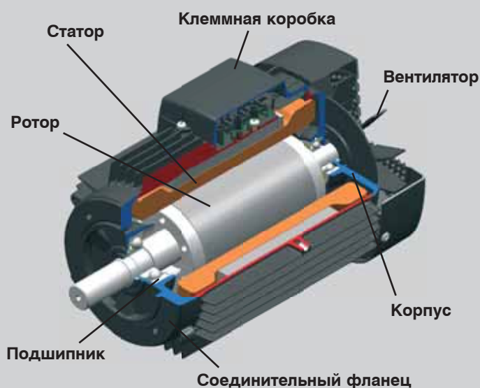
Электродвигатель
