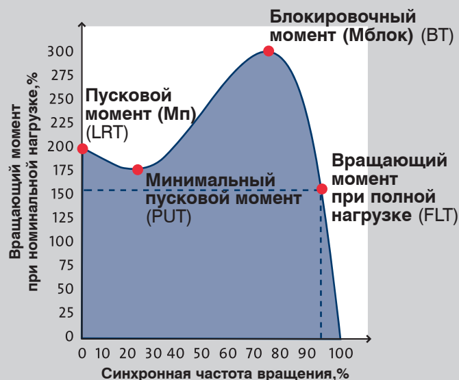
Характеристика вращающий момент/частота вращения для электродвигателя переменного тока
