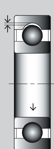
Радиальный внутренний зазор
