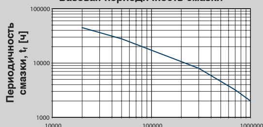
Величина подшипника (мм/мин)
