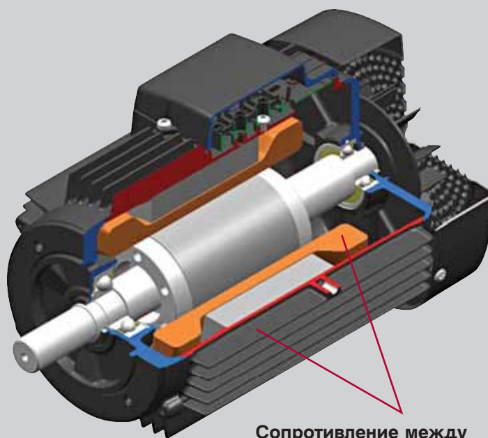
Сопротивление между обмотками и корпусом
