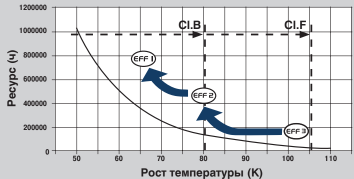
Зависимость ресурса от температуры
