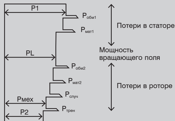
Схема, отображающая потери в электродвигателе
