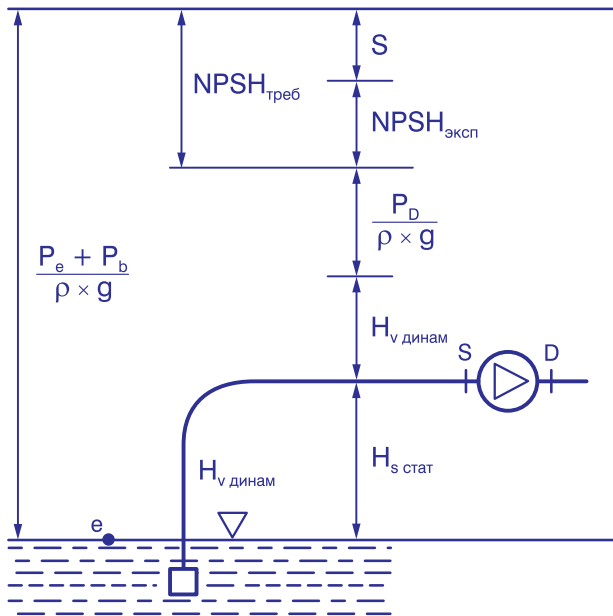
Рис. 16. Всасывание насоса.
