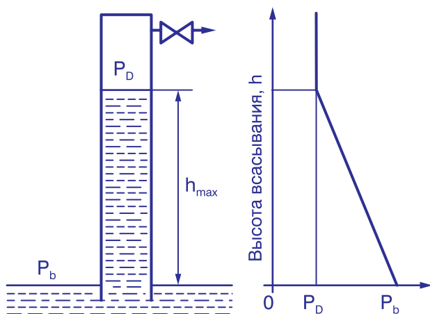
Рис. 15. Давление на стенки трубы h_{max}
