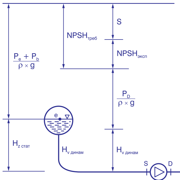
Рис. 17. Нагнетание насоса.
